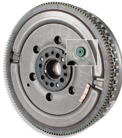
Fig. 1: De transportborging wordt bij de eerste start binnen in het tweedelig vliegwiel afgebroken
