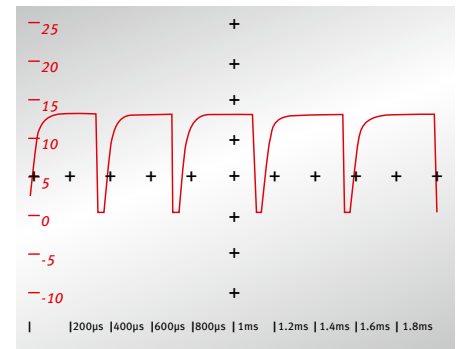
Signal bei Leerlauf (abhängig von Leerlaufdrehzahl)
