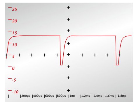
Signal bei Gasstoß
