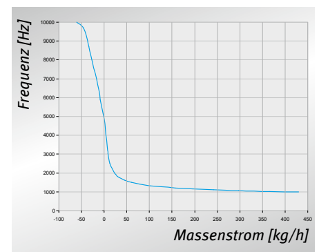
Kennlinie Massenströmsensor
