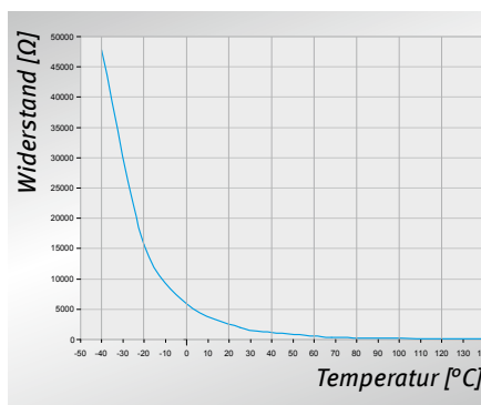
Kennlinie Temperatursensor
